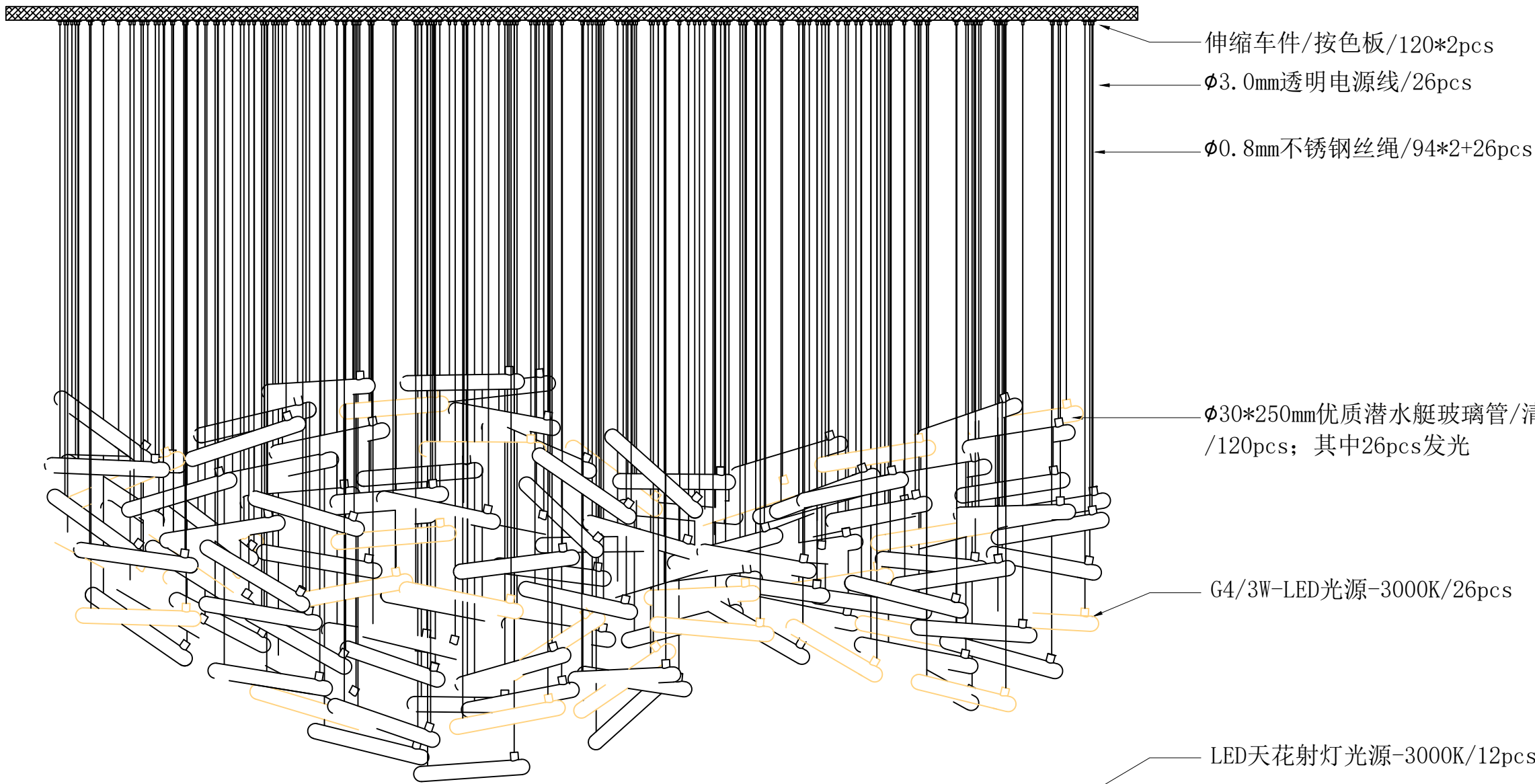
主视图
